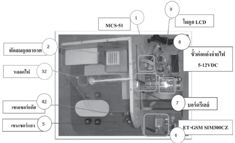
รูปที่ 5 ส่วนประกอบของโมดูลห้องครัวจำลอง
