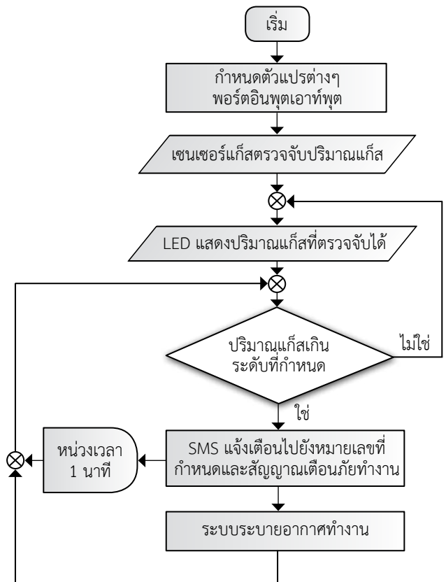
รูปที่ 1 แผนผังโปรแกรมของระบบการตรวจจับปริมาณก๊าซแอลพีจีพร้อมระบบส่งสัญญาณเตือนภัย
